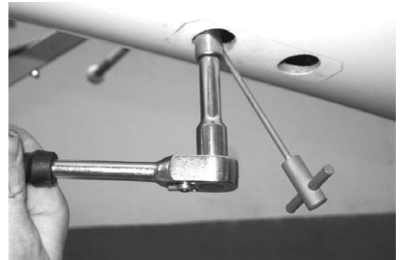
Herausschrauben der Zündkerze, Werkzeug bleibt auf Stecker aufgefädelt
