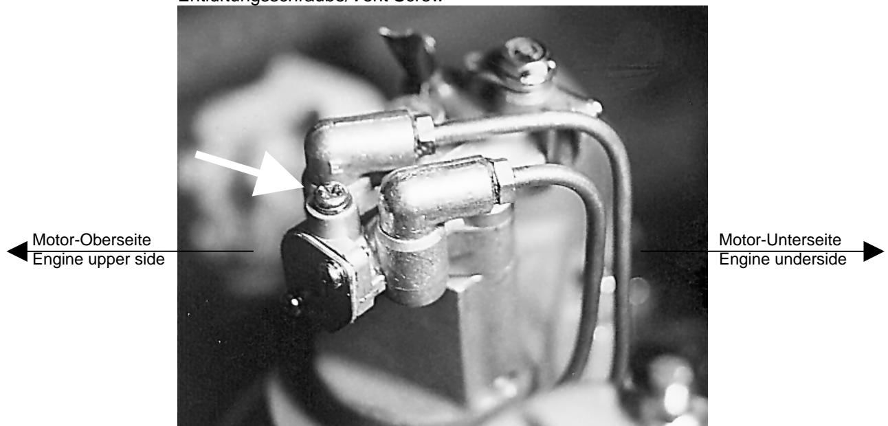
Entlüftungsschraube/Vent Screw
